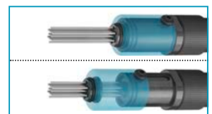
Nastavitelné jehlové saně s integrovaným vedením jehly zaručují dlouhou životnost
